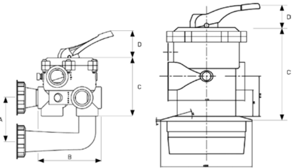
Vari-Flo™ szelep SP0719SKR-LP (a csatlakozók külön vásárolhatók)
